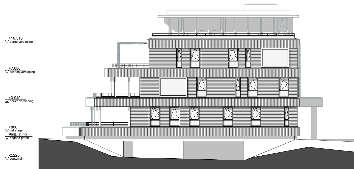
Gevelaanzicht Zuid
