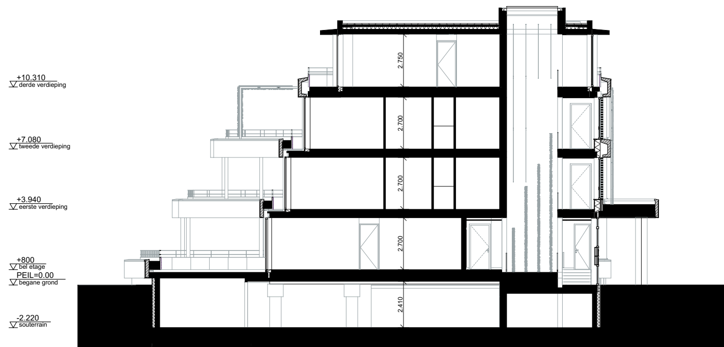
Doorsnede A
